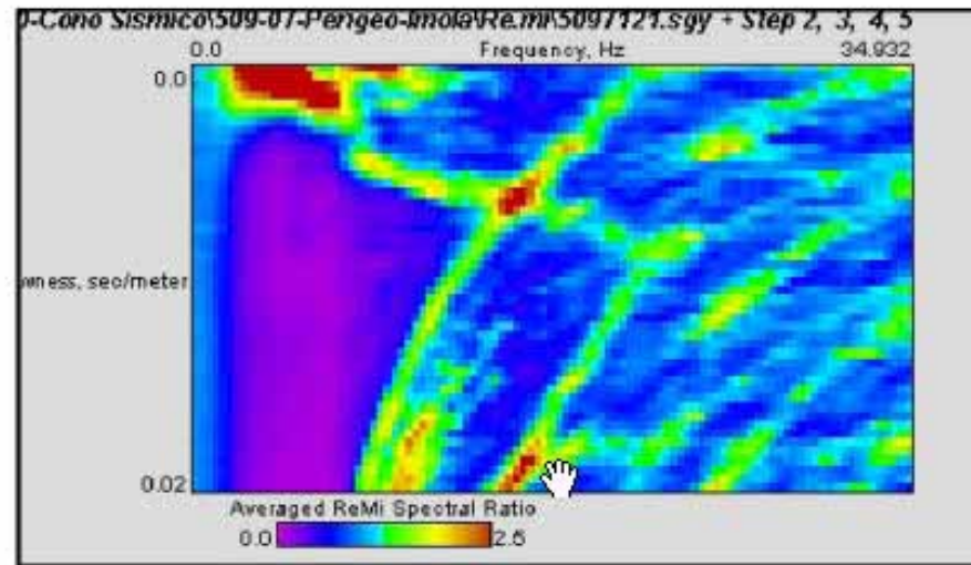
Curva di dispersione
