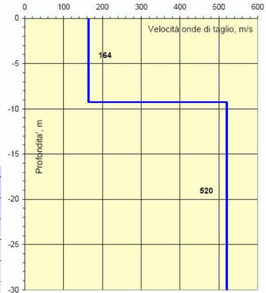
MODELLO DI VELOCITA' ONDE DI TAGLIO - Sezione -
