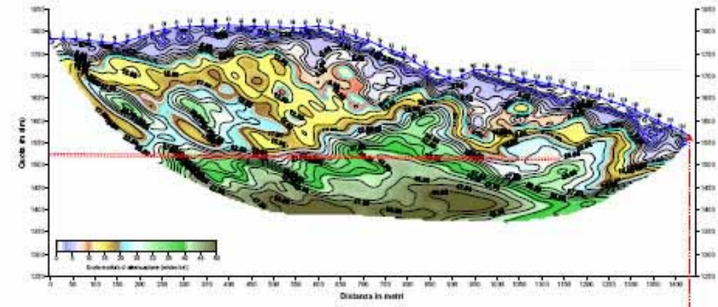
SEZIONE SISMICA TOMOGRAFICA 11 [Modulo di Attenuazione]
