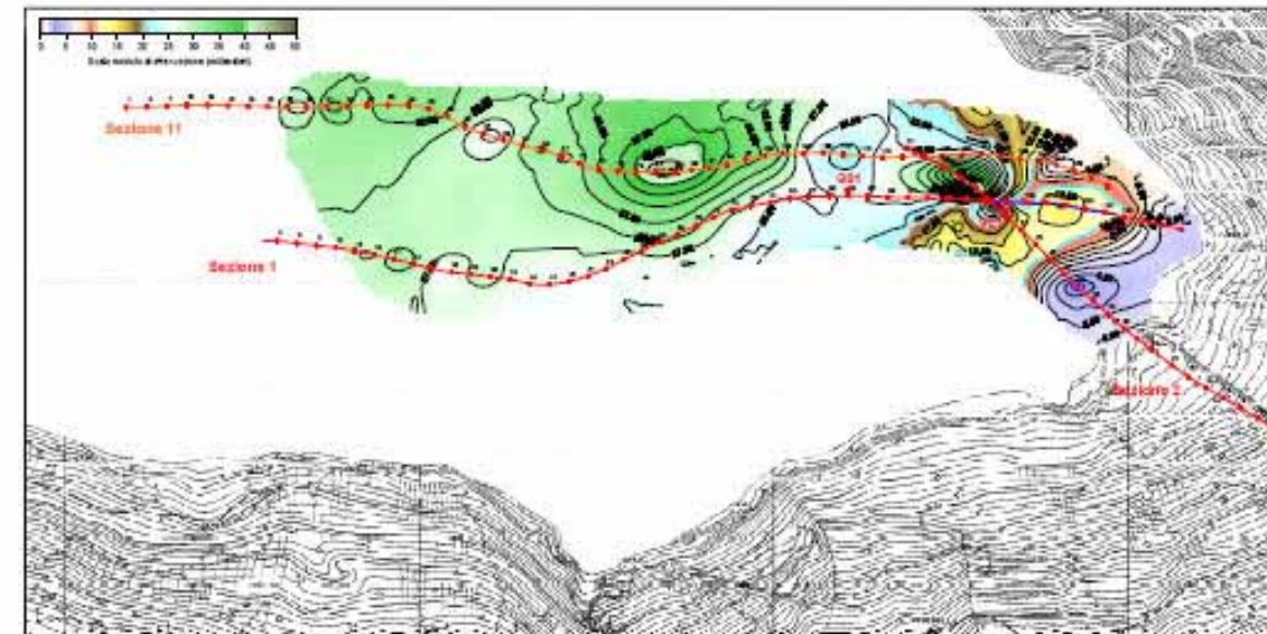
SLICE IN MODULO DI ATTENUAZIONE SEZIONE PLANARE ALLA QUOTA DI 1515-1520 M SLM QUOTA DELLA GALLERIA IDRAULICA
