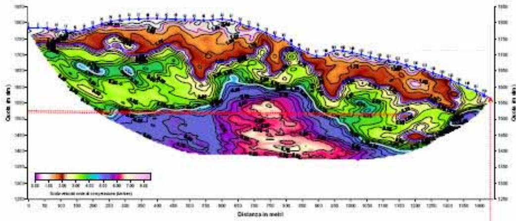
SEZIONE SISMICA TOMOGRAFICA 11 [Velocità onde di compressione]
