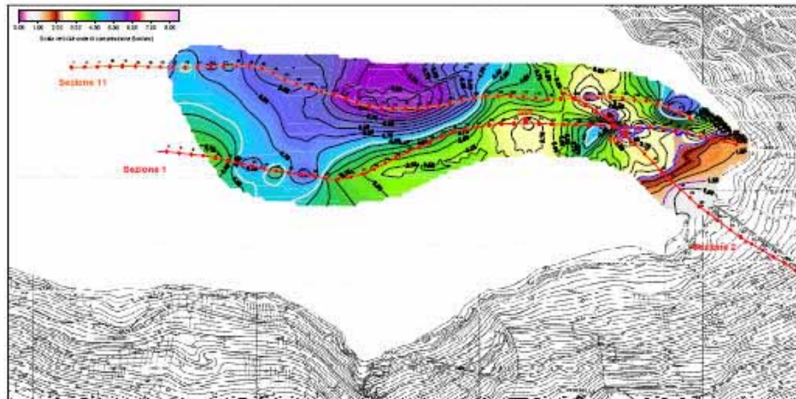
SLICE IN VELOCITA' DELLE ONDE DI COMPRESSIONE SEZIONE PLANARE ALLA QUOTA DI 1515-1520 M SLM QUOTA DELLA GALLERIA IDRAULICA
