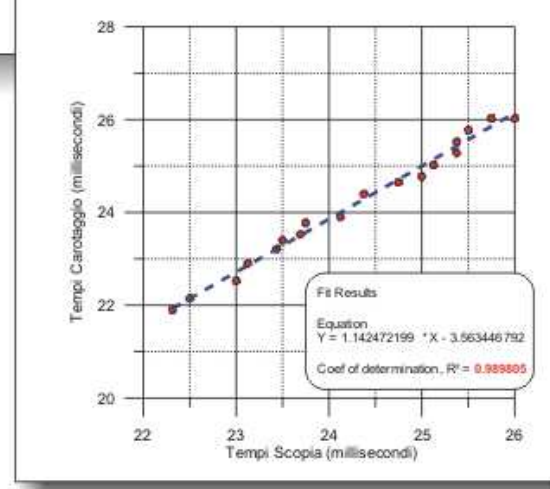
FIT DATI DA -51.0 A -59.5 M DAL P.C. SCOPIA PARATIA - CAROTAGGIO TERRENO
